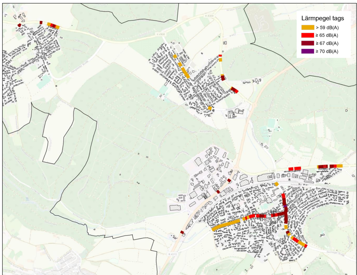
Abbildung 6: Pegelüberschreitungen im Tageszeitraum
